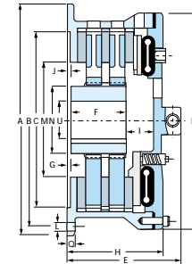
LIM Clutch/Kupplung (LIM 108-LIM 242)
