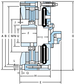
LIM 106 Clutch/Kupplung
