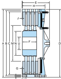
LIM 360 Clutch/Kupplung
